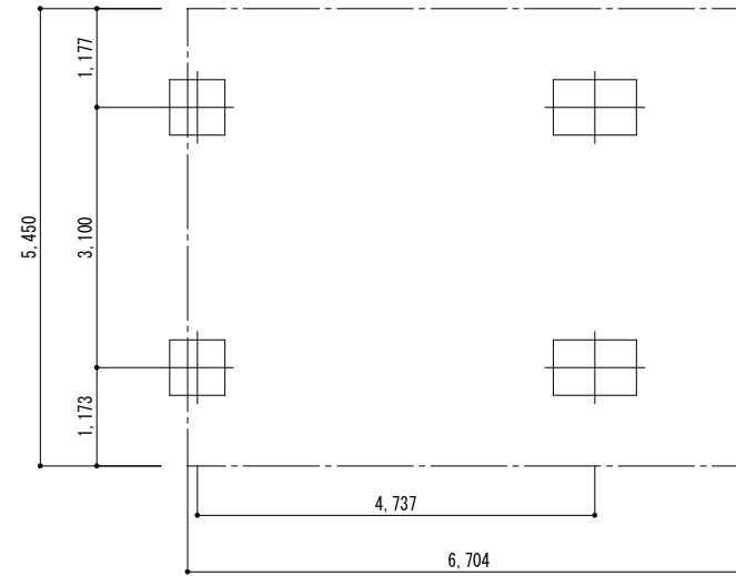
■基礎配置図
